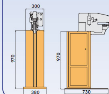
Basamento fisso (mm) Fixed Stand
